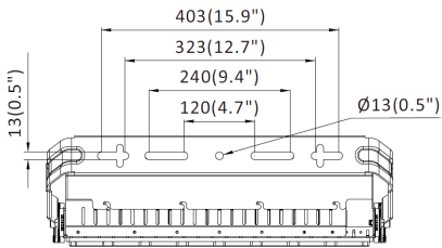
Bracket(480W-1500W)
